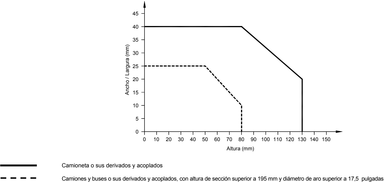
Figura 19. Daños en el área de los costados, tamaño máximo a reparar
